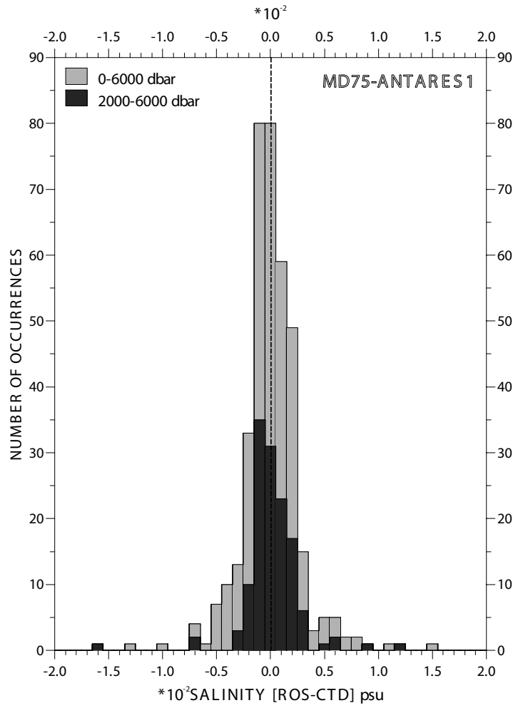
Histogramme des delta SALINITE
