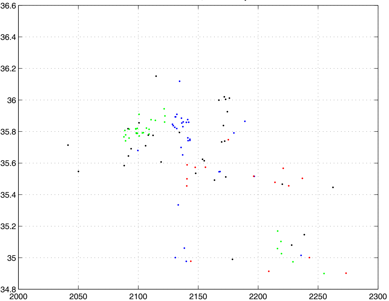
TCO2 out en x, salinité en y
