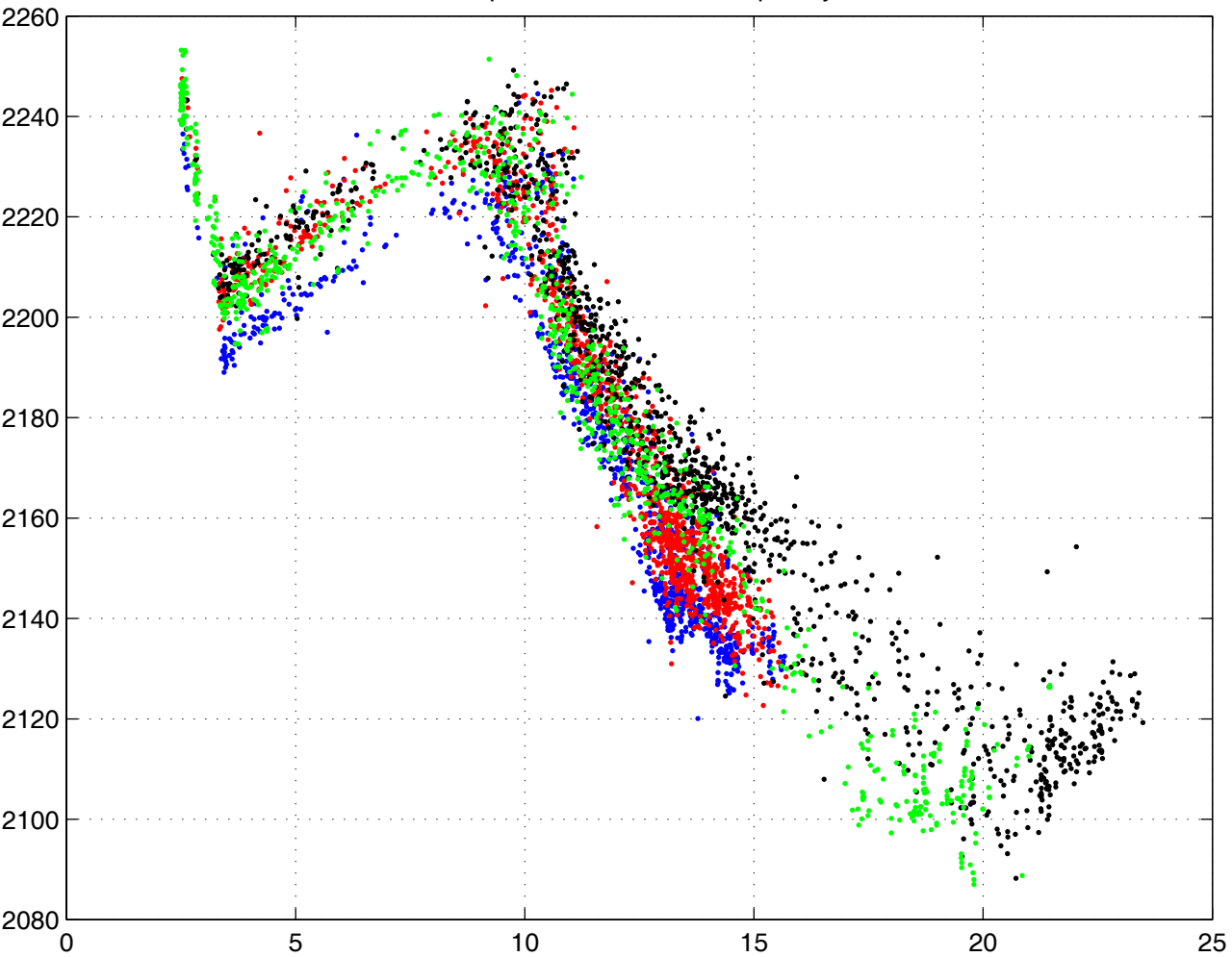
température en x, TCO2 kept en y
