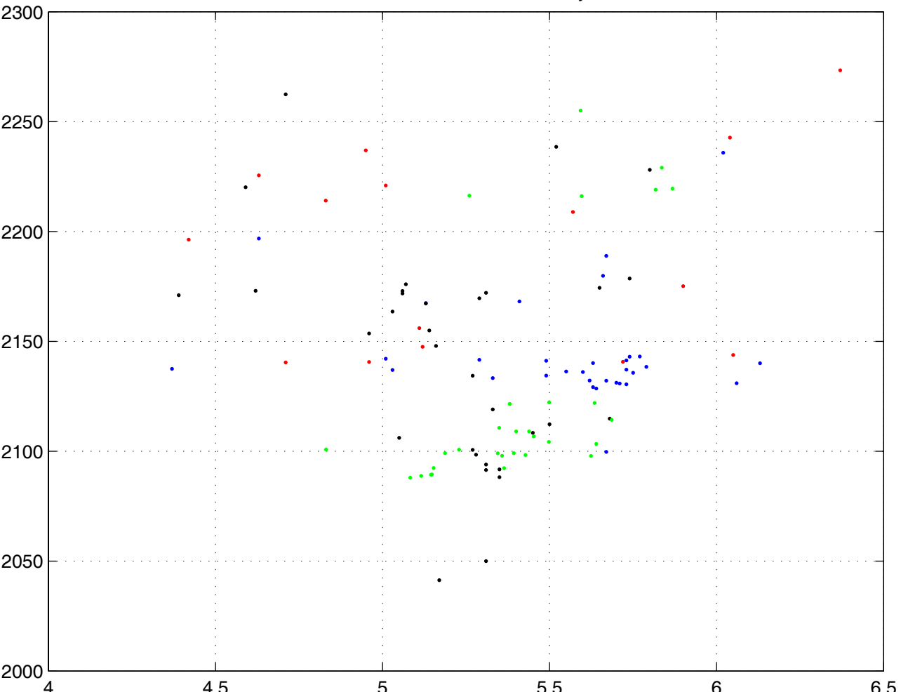
O2 CTD en x, TCO2 out en y
