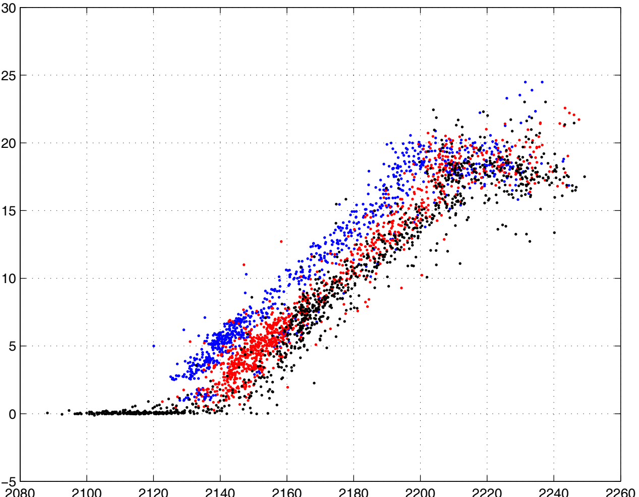
TCO2 kept en x, NO3 en y
