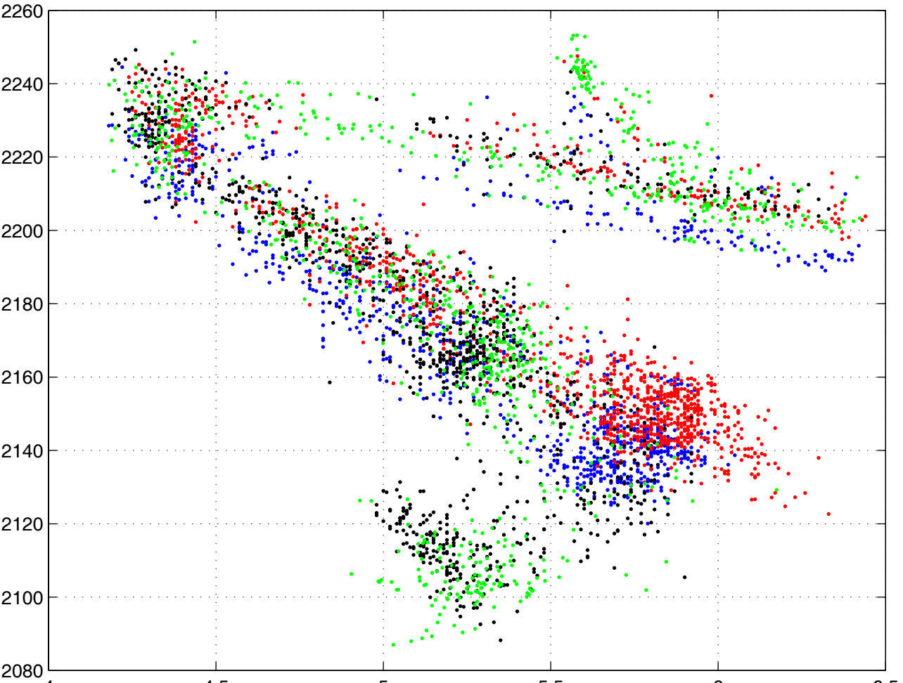
O2 CTD en x, TCO2 kept en y
