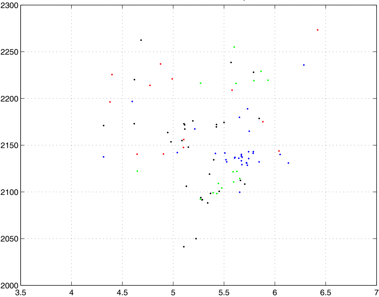
Oxidos en x, TCO2 out en y
