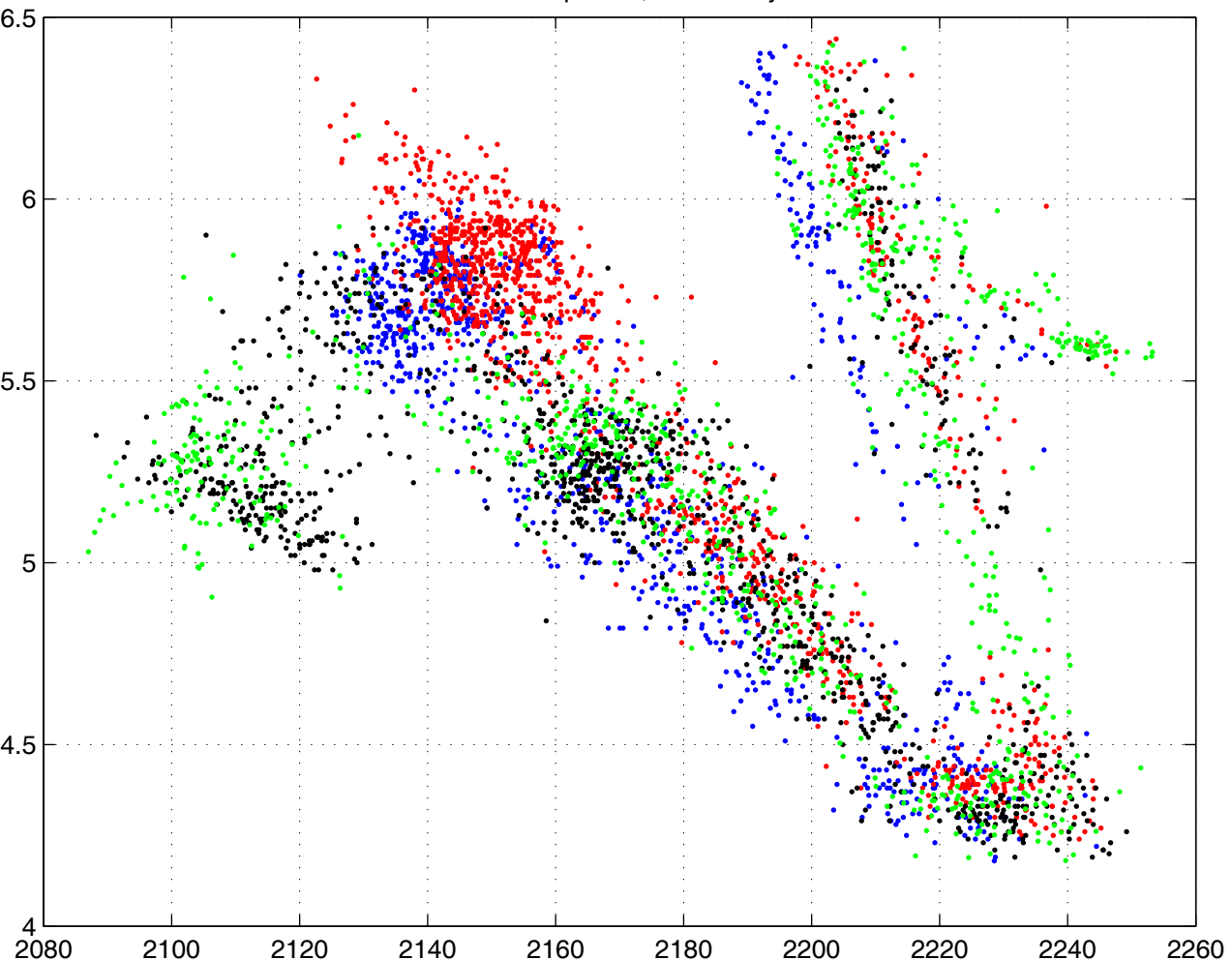
TCO2 kept en x, O2ctd en y
