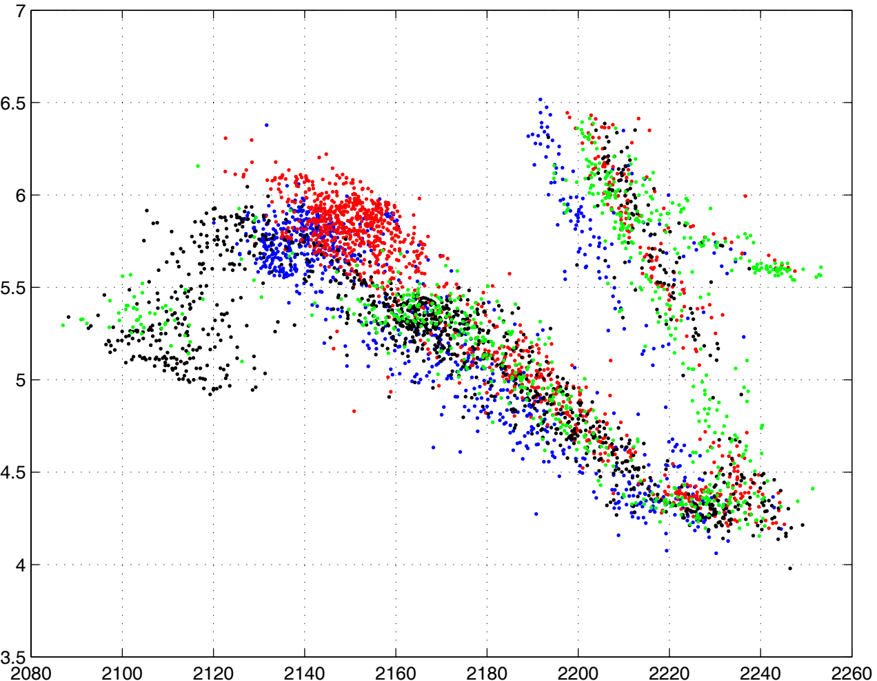
TCO2 kept en x, oxdos en y
