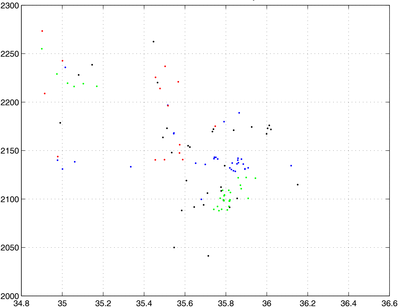
salinité en x, TCO2 out en y
