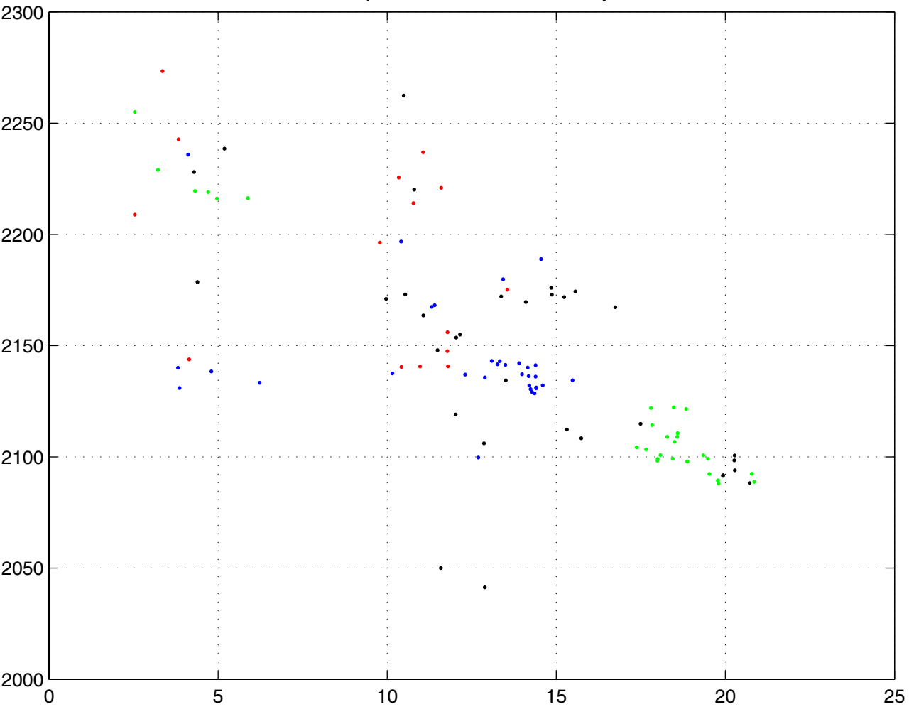
température en x, TCO2 out en y
