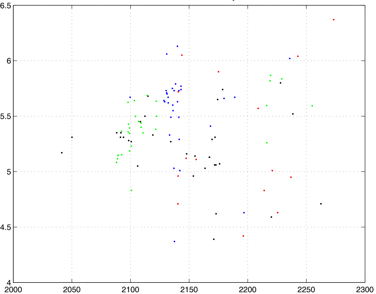
TCO2 out en x, O2ctd en y
