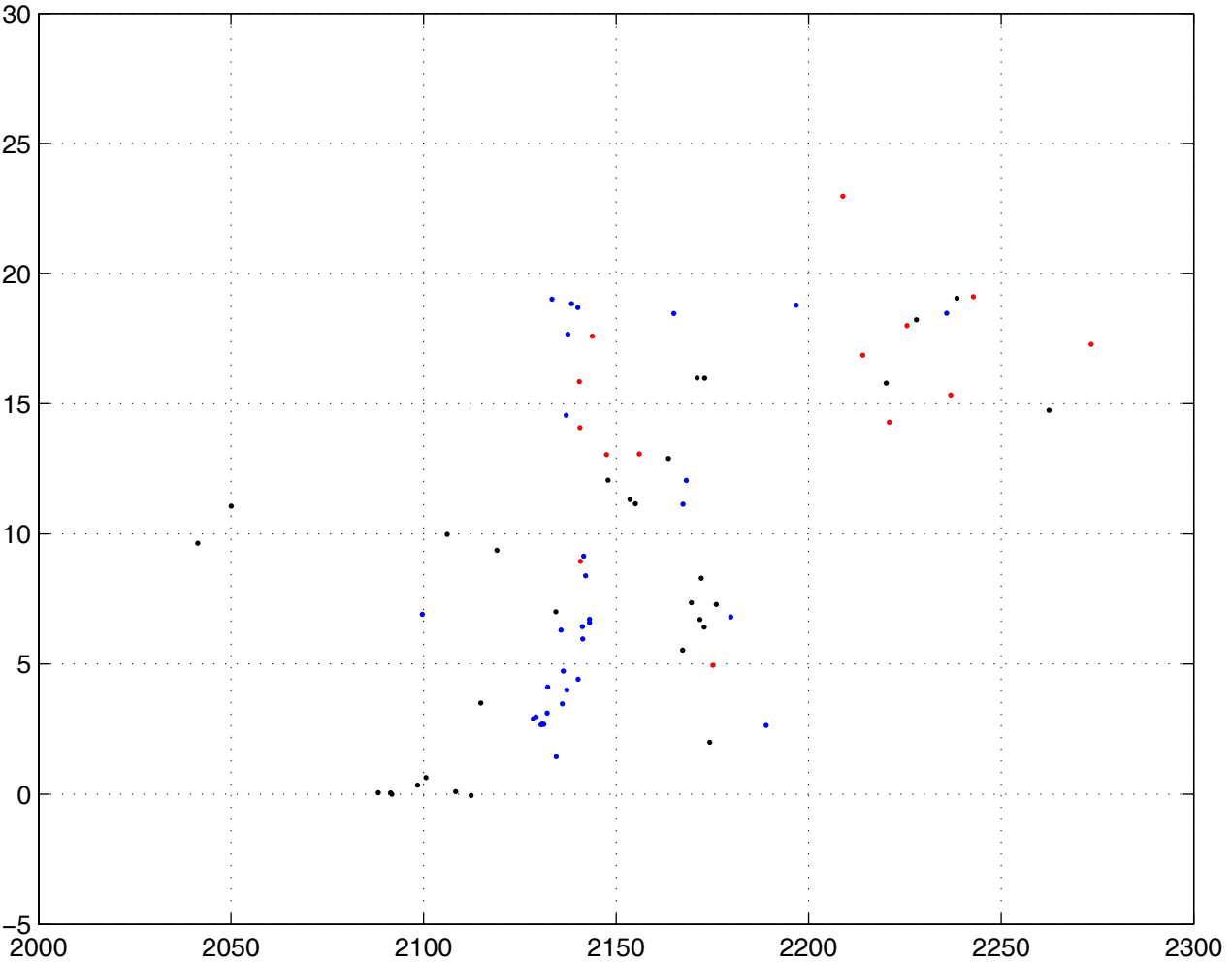
TCO2 out en x, NO3 en y
