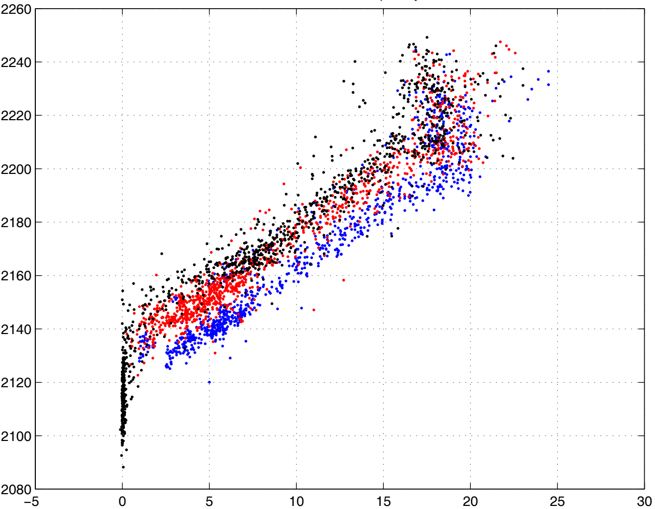
NO3 en x, TCO2 kept en y
