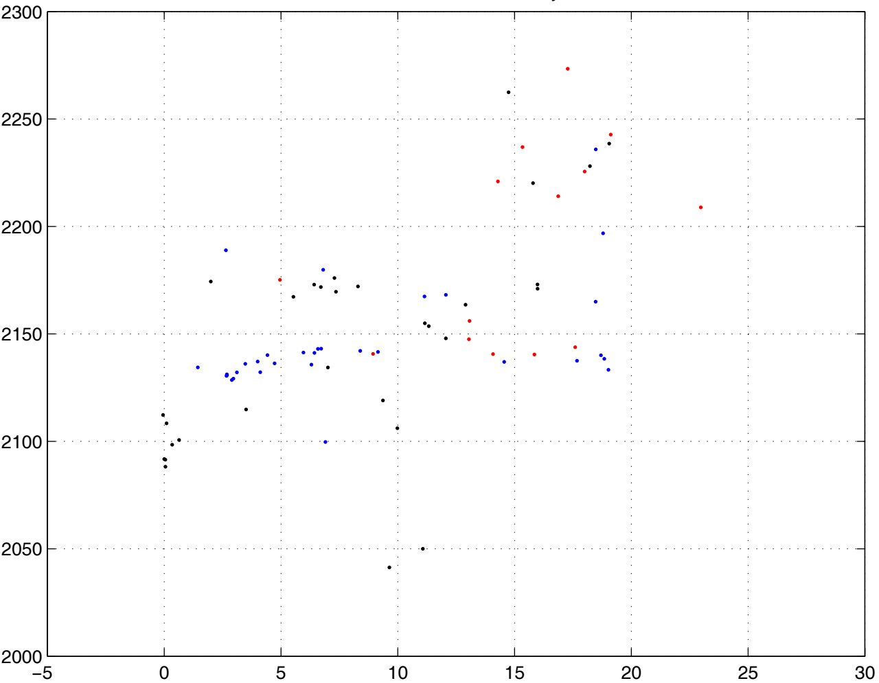
NO3 en x, TCO2 out en y
