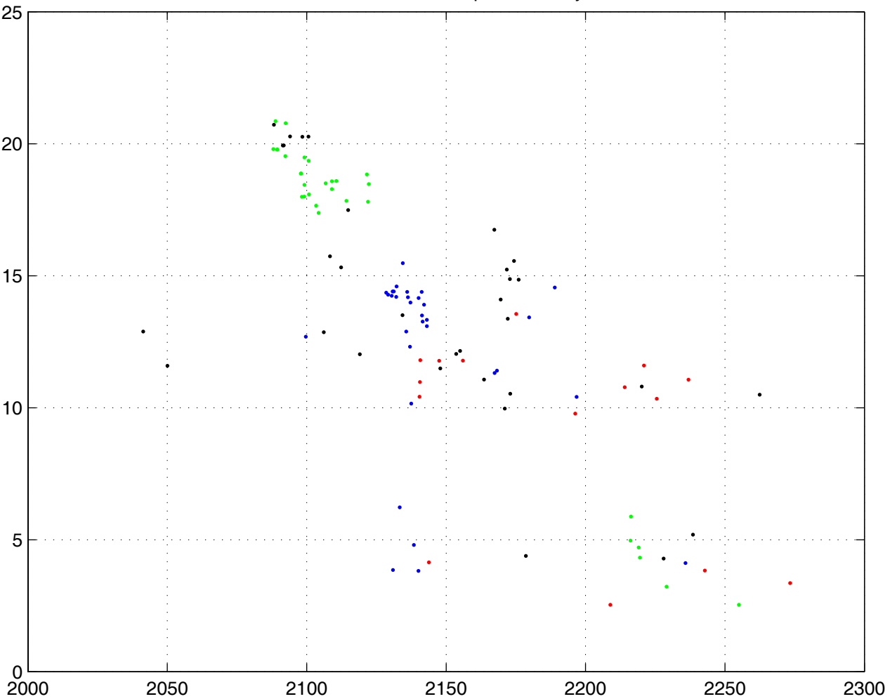
TCO2 out en x, température en y
