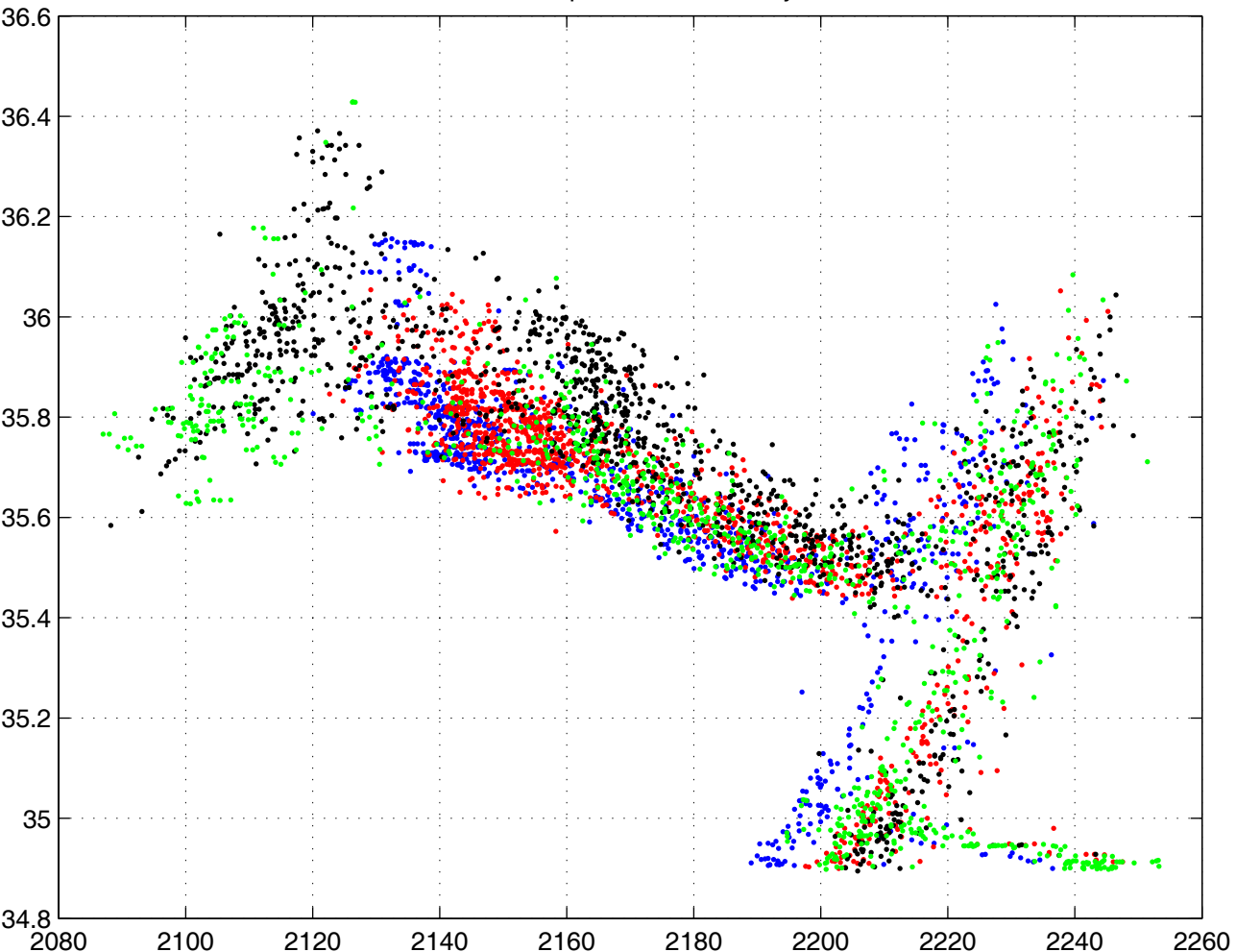
TCO2 kept en x, salinité en y
