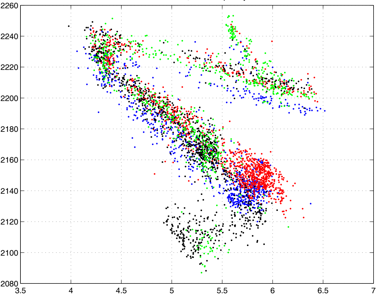
Oxdos en x, TCO2 kept en y
